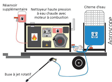
Remorque avec nettoyeur et citerne d'eau assemblés.
